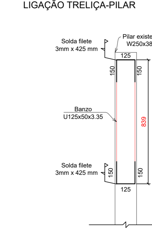
DETALHE 2 LIGAÇÃO TRELÇA-PILAR
