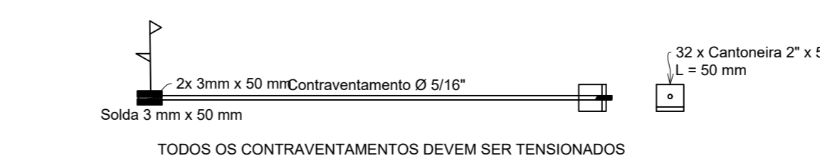
DETALHAMENTO CONTRAVENTAMENTO
