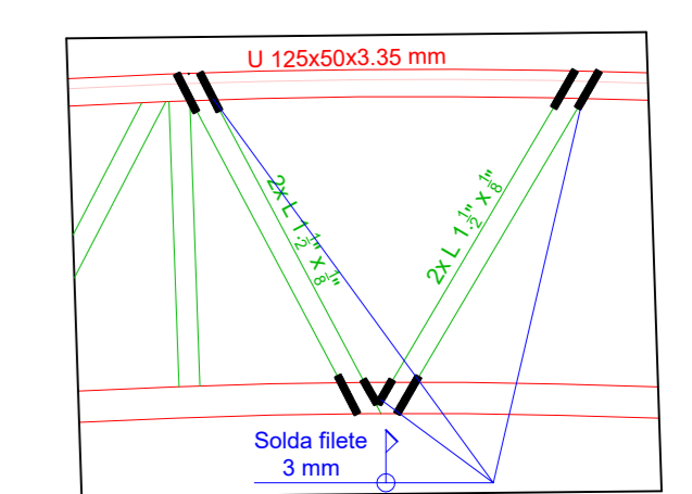
DETALHE 4 SOLDA DIAGONAIS
