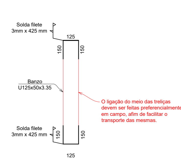
DETALHE 3 LIGAÇÃO MEIO TRELÇA-TRELÇA
