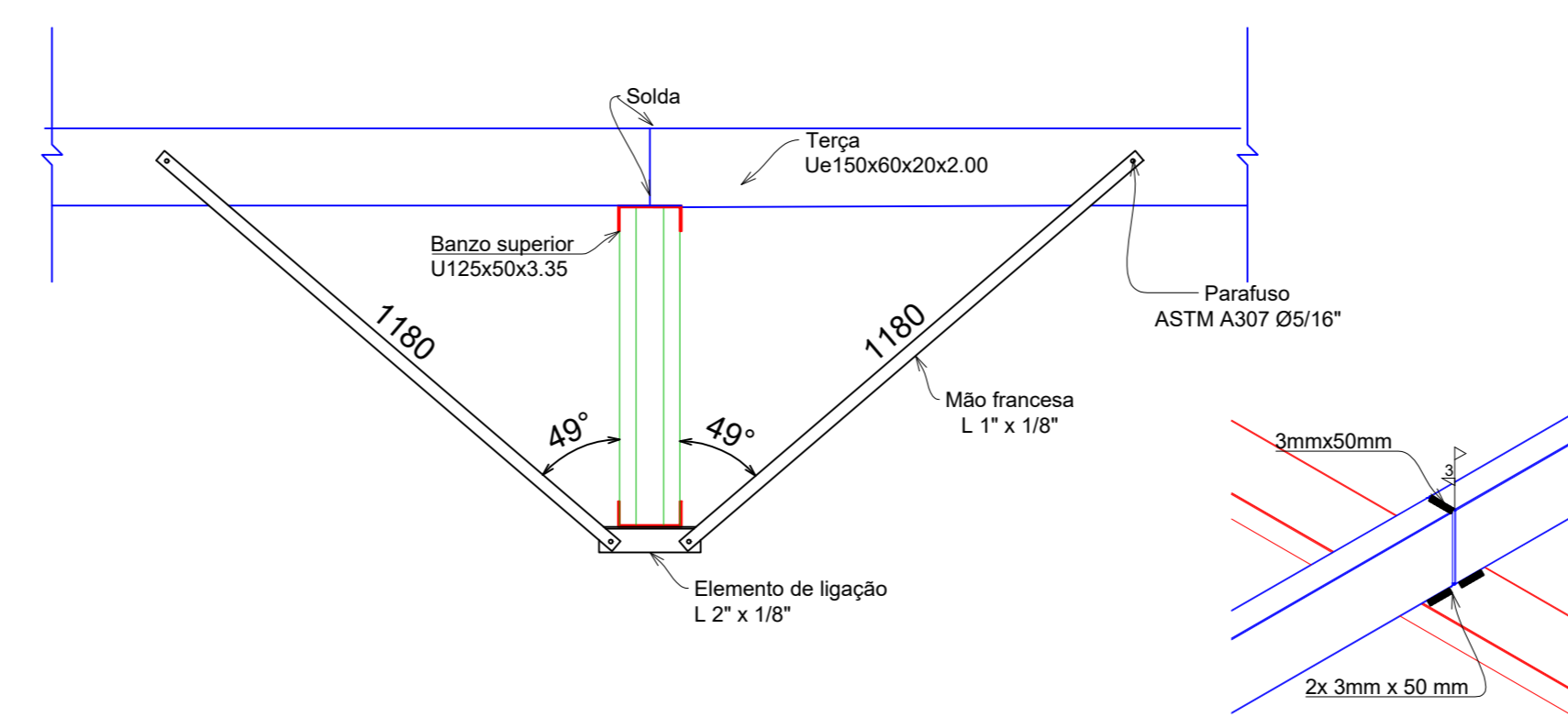
DETALHE 1 LIGAÇÃO MÃO-FRANCA / TRELIÇA-TERÇA
