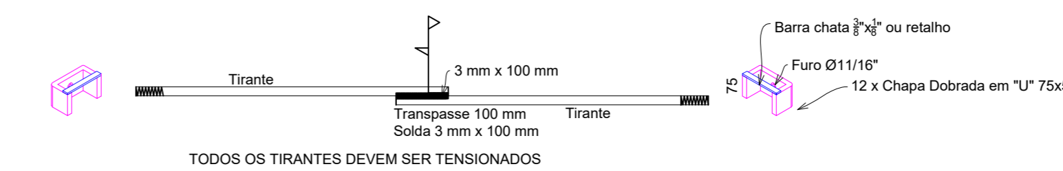
DETALHAMENTO CONTRAVENTAMENTO
